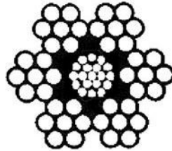
6 X 7 + 1 X 19 Mermer Halatı
