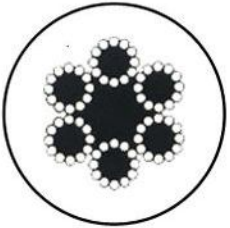
İzoleli Halat (PVC Kaplı)
