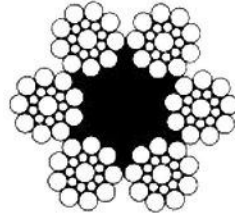
6 X 19S Gırgır Halatı
