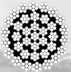
36 X 7 Nufleks Halat Galvanizli
