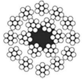
18 X 7 Dönmez Halat
