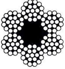
6 X 19 L. ÖZ Siyah / Galvanizli
