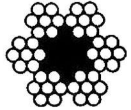
6 x 7 L. ÖZ Galvanizli
