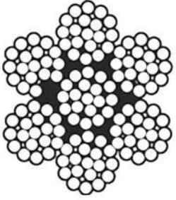
7 x 19 Krom Halat (Inox)
