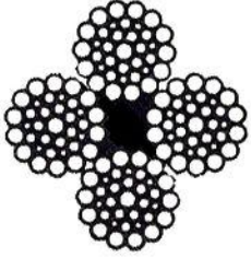
4 X 26 Trifor Halatı
