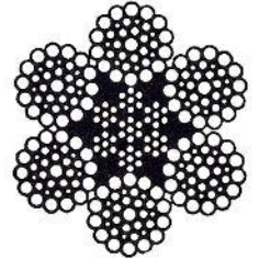
6 x 26 Ç. ÖZ / L. ÖZ Siyah
